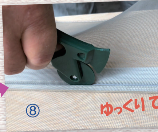
⑧ 端部からクリップで押さえ、ワンタッチローラーで溝へ押し込みます。
