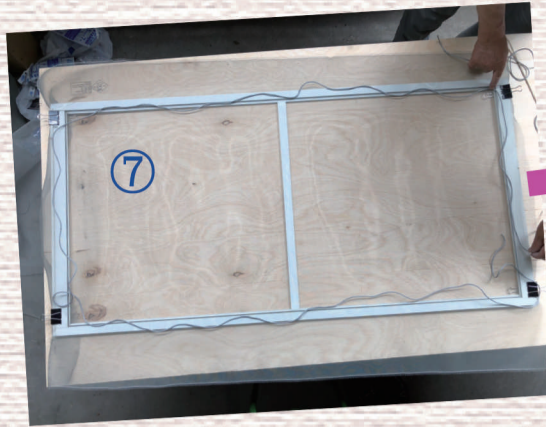
⑦ 新しい押さえゴムを網戸の溝にそって配置します。
